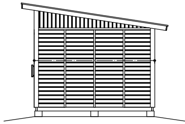
OIKEALTA
