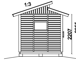
VASEMMALTA
