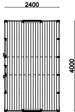
POHJA
