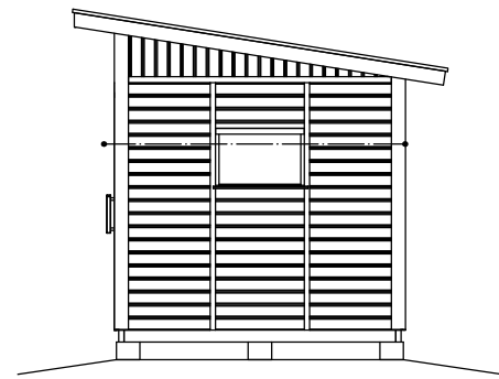
OIKEALTA
