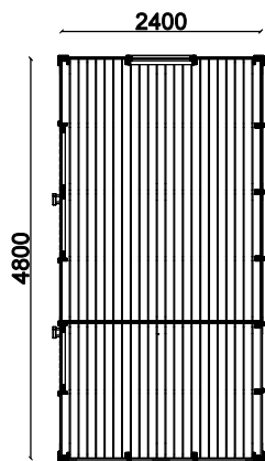
POHJA
