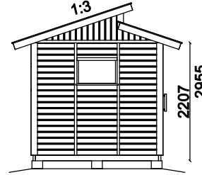
VASEMMALTA
