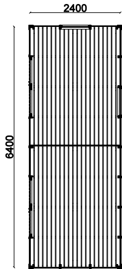
POHJA
